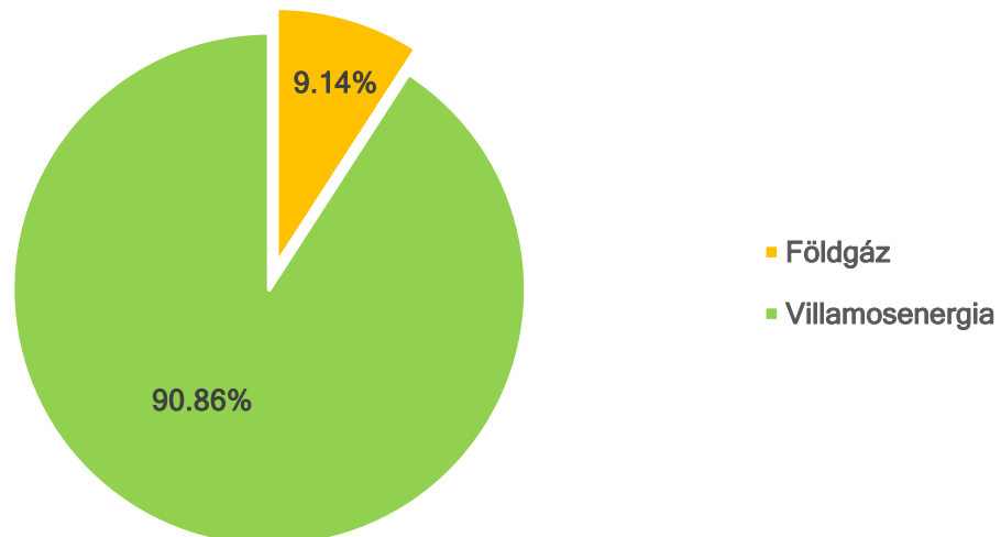
2. ábra A szén-dioxid kibocsátás megoszlása az energiahordozók között
